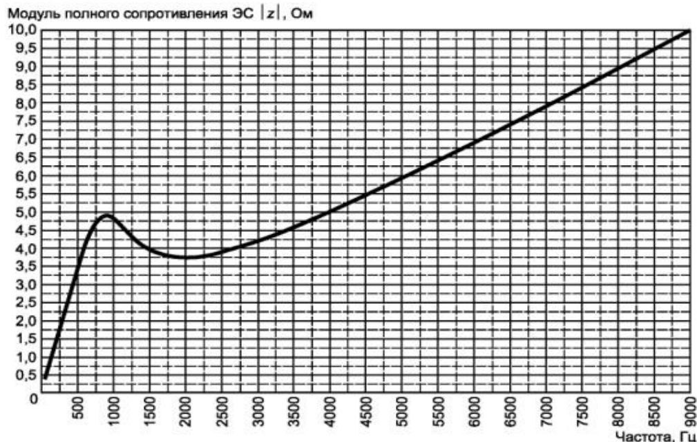
Рисунок В.5 - Модуль полного сопротивления эквивалента сети
