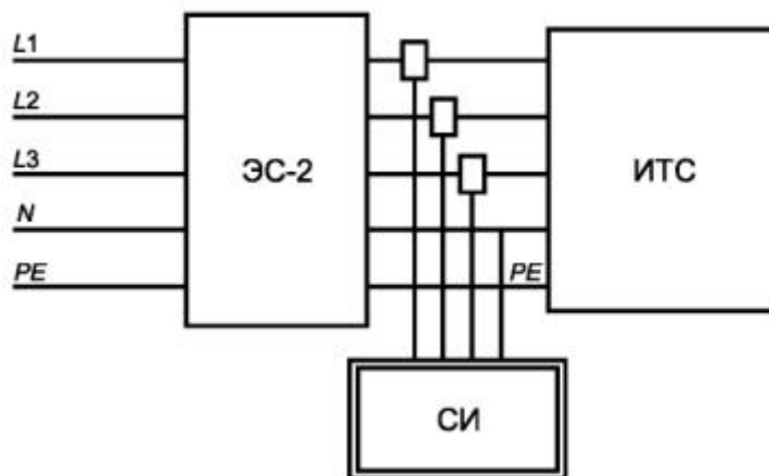
Рисунок В.2 - Схема измерений эмиссии составляющих потребляемого тока ТС в однофазных системах
