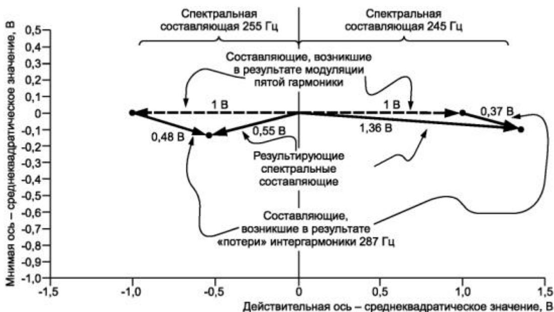
Рисунок С.7 - Векторы спектральных составляющих, их на частотах 245 и 255 Гц
