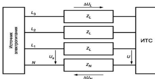
Рисунок 2 - Схема измерений эмиссии в однофазных системах
